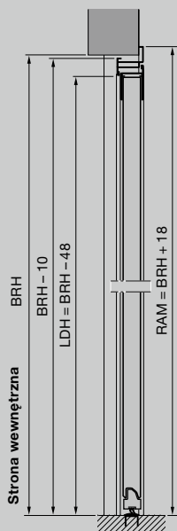
Drzwi boczne z aluminiową ościeżnicą kątową, profil typu 2 Mocowanie na zewnątrz
