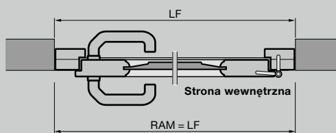
Drzwi boczne z litego drewna Montaż w otworze
